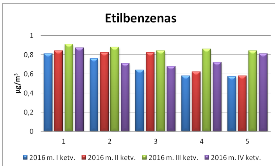
9 pav. 2016 m. Etilbenzeno koncentracijos vizualizacija Pakruojo rajone.
