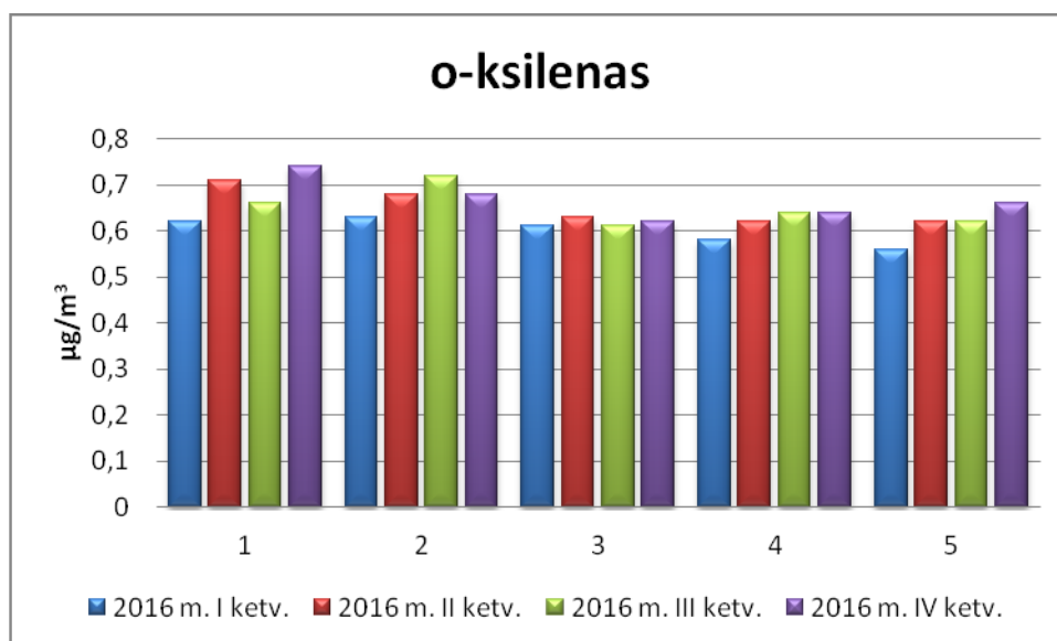
11 pav. 2016 m. O-ksileno koncentracijos vizualizacija Pakruojo rajone.
