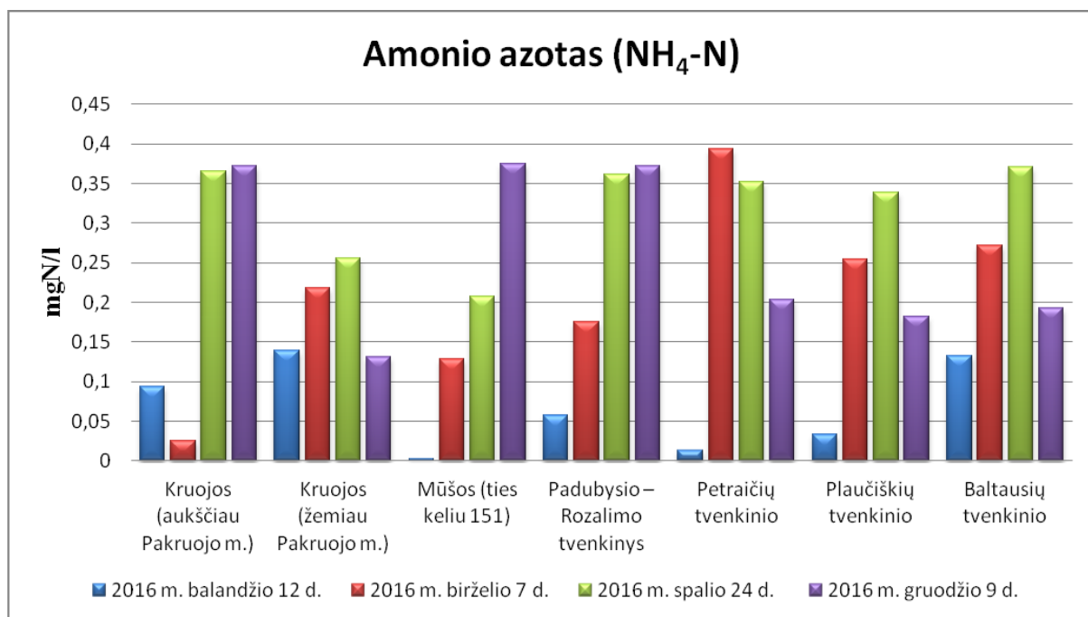
19 pav. \text{NH}_4\text{-N} koncentracija Pakruojų rajono paviršiniuose vandens telkiniuose.
