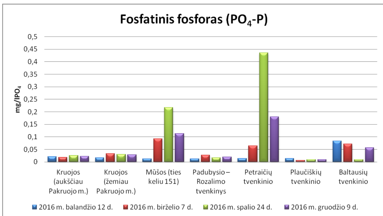
20 pav. \text{PO}_4\text{-P} koncentracija Pakruojų rajono paviršiniuose vandens telkiniuose.
