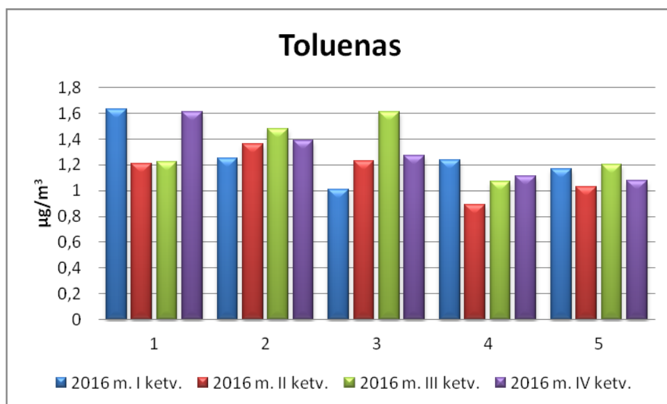
8 pav. 2016 m. Tolueno koncentracijos vizualizacija Pakruojo rajone.
