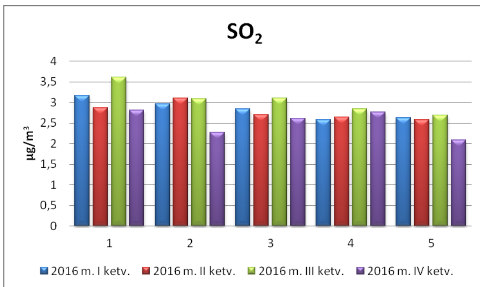
6 pav. 2016 m. SO 2 koncentracijos vizualizacija Pakruojo rajone.
