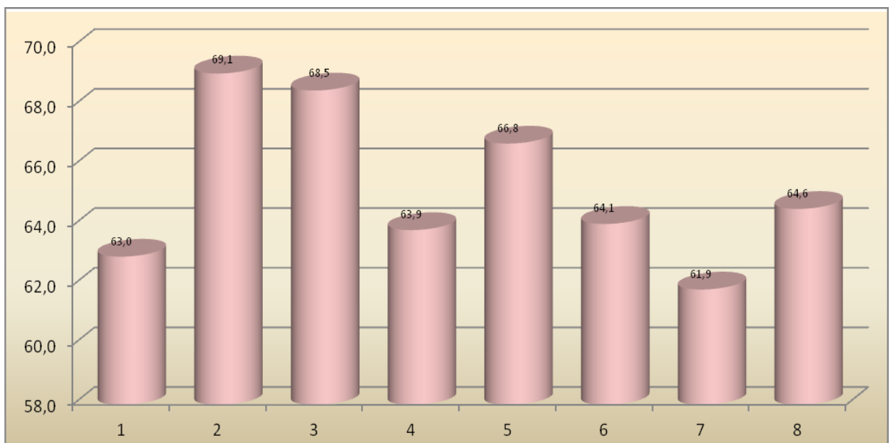
54 pav. Maksimalaus triukšmo pasiskirstymas matavimo vietose vakaro metu (18-22val.). Ribinis dydis 65 dBA.
