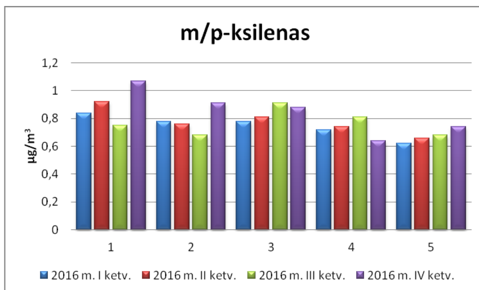
10 pav. 2016 m. M/p ksileno koncentracijos vizualizacija Pakruojo rajone.
