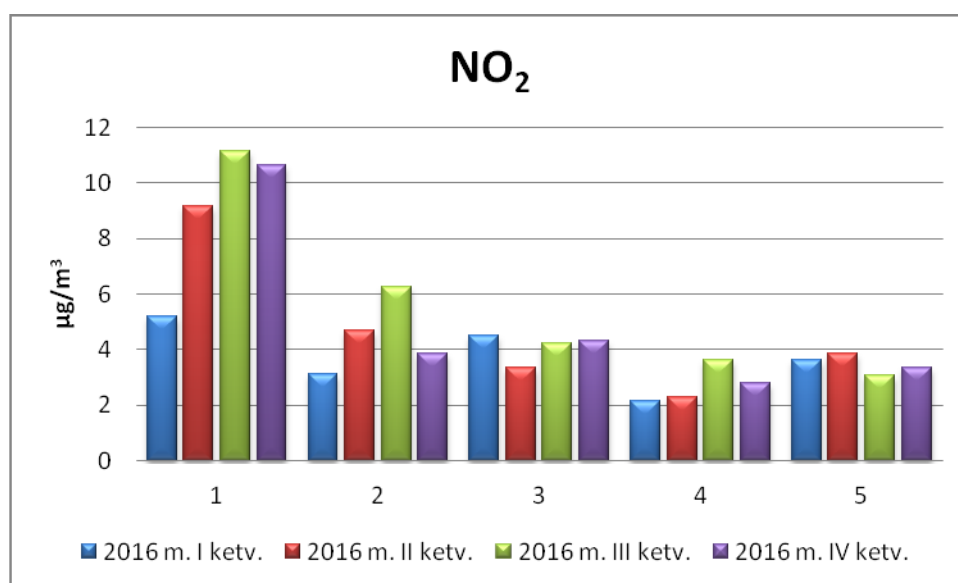
5 pav. 2016 m. NO 2 koncentracijos vizualizacija Pakruojo rajone.
