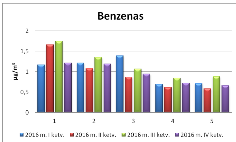
7 pav. 2016 m. Benzeno koncentracijos vizualizacija Pakruojo rajone.
