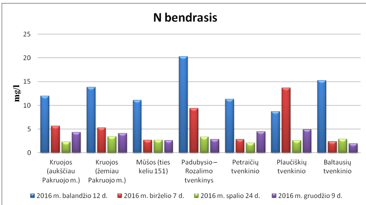
21 pav. N_b koncentracija Pakruojų rajono paviršiniuose vandens telkiniuose.
