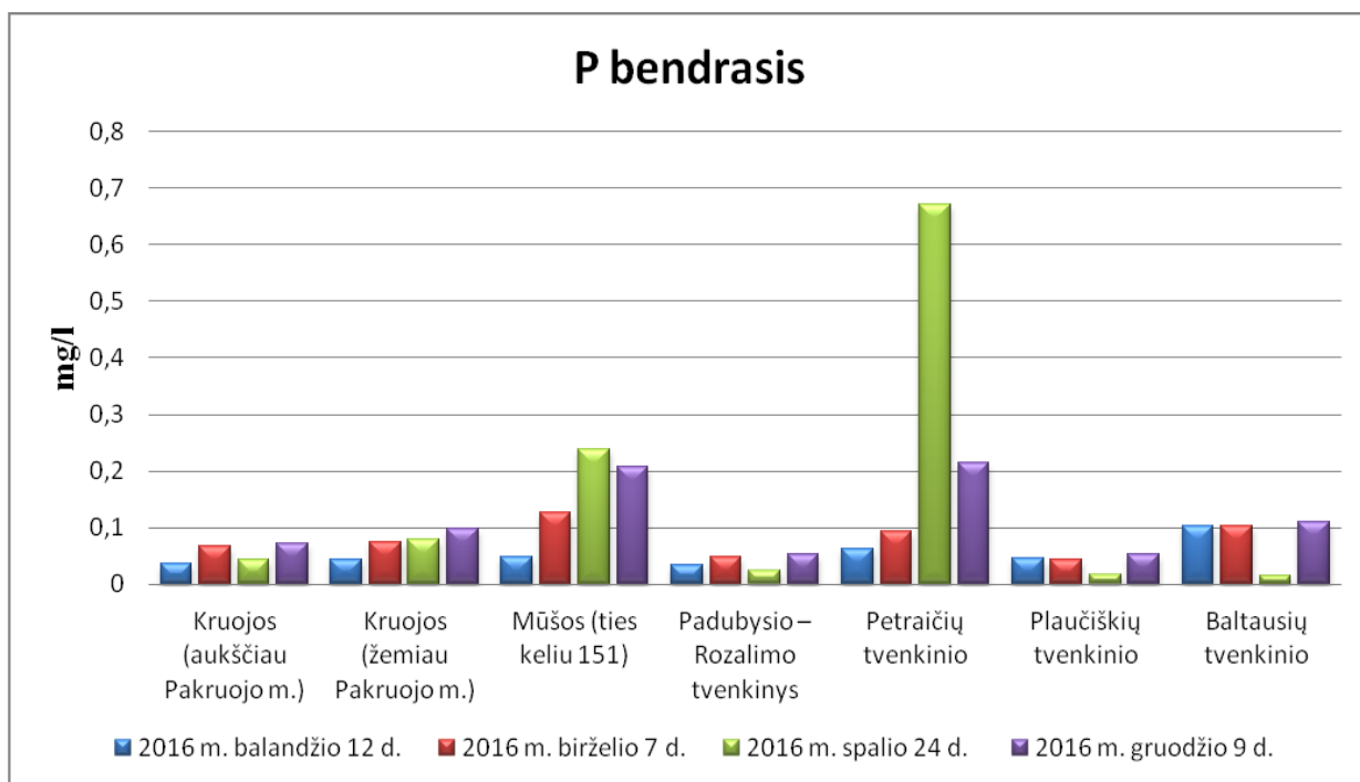
22 pav. P_b koncentracija Pakruojų rajono paviršiniuose vandens telkiniuose.
