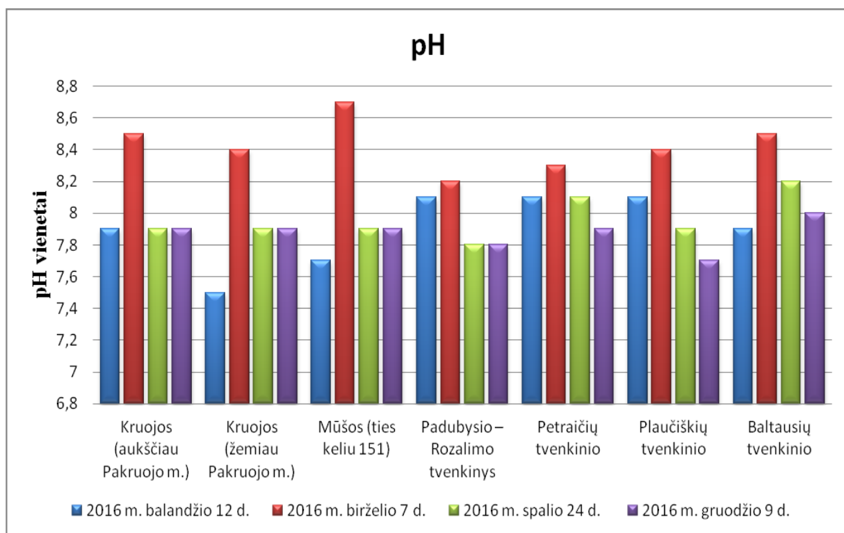
14 pav. pH vienėtų skaičius Pakruojos rajono paviršiniuose vandens telkiniuose.
