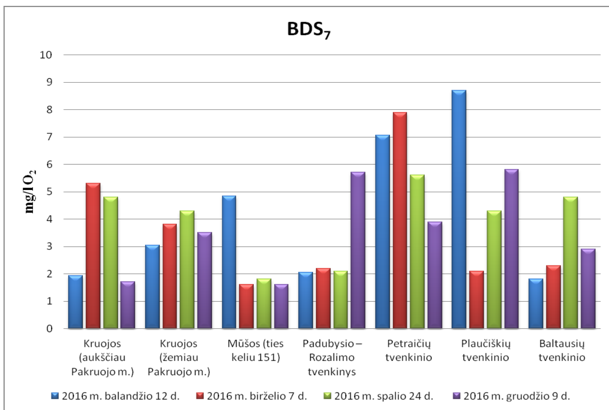
16 pav. BDS 7 koncentracija Pakruojos rajono paviršiniuose vandens telkiniuose.
