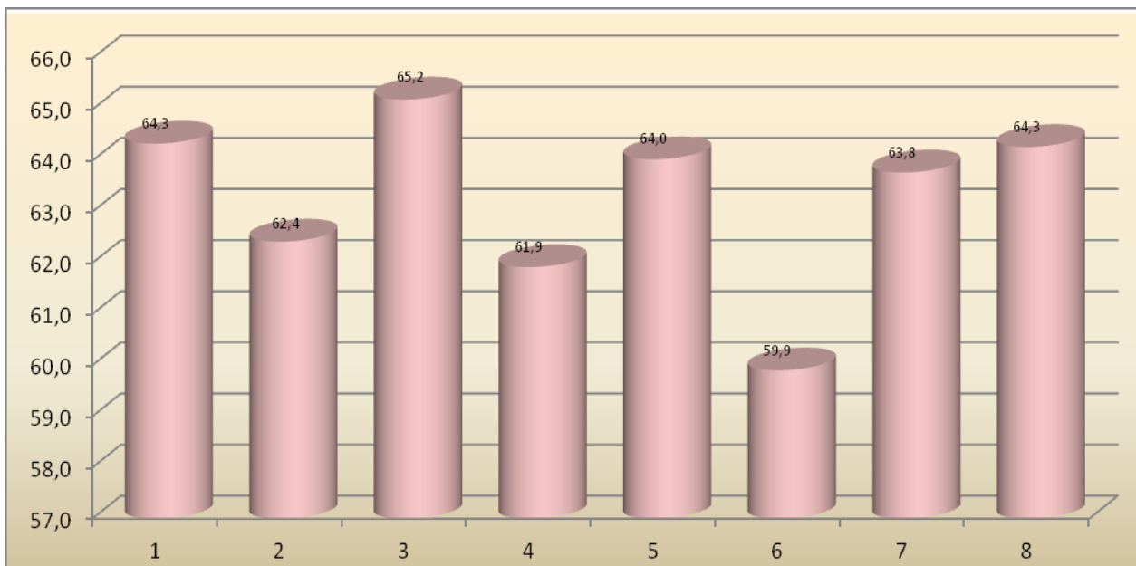
38 pav. Maksimalaus triukšmo pasiskirstymas matavimo vietose vakaro metu (18-22val.). Ribinis dydis 65 dBA.
